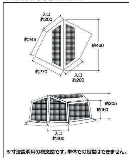
平面図・設営時寸法(単位 cm)
